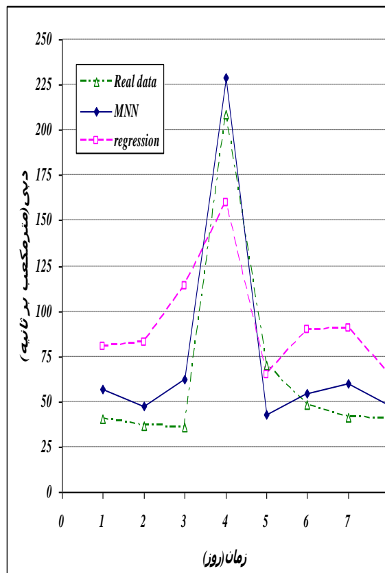
شکل شماره ۱۲- مقایسه هیدروگراف سیل خروجی و روندیابی شده با مدل های مختلف مربوط به سیلاب بهمن ماه ۱۳۸۰
