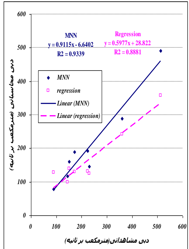
شکل شماره ۸- مقایسه مقادیر دبی مشاهده‌ای و محاسباتی حاصل از روندیابی هیدروگراف سیل با مدل‌های مختلف به ازای سیل دی ماه ۱۳۸۰
