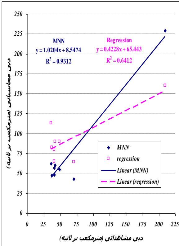
شکل شماره ۹- مقایسه مقادیر دبی مشاهده‌ای و محاسباتی حاصل از روندیابی هیدروگراف سیل با مدل‌های مختلف به ازای سیلاب بهمن ماه ۱۳۸۰
