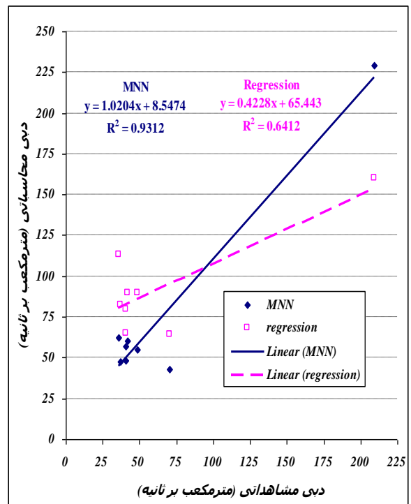
شکل شماره ۱۰- مقایسه مقادیر دبی مشاهده‌ای و محاسباتی حاصل از روندیابی هیدروگراف سیل با مدل‌های مختلف به ازای سیلاب فروردین ماه
