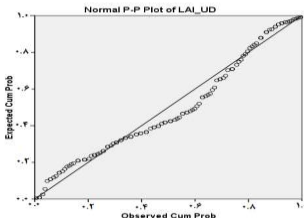
شکل ۳: p-p plot جهت بررسی نرمال بودن توزیع داده‌های شاخص سطح برگ Figure 3: P-p plot to study the distribution of LAI data
