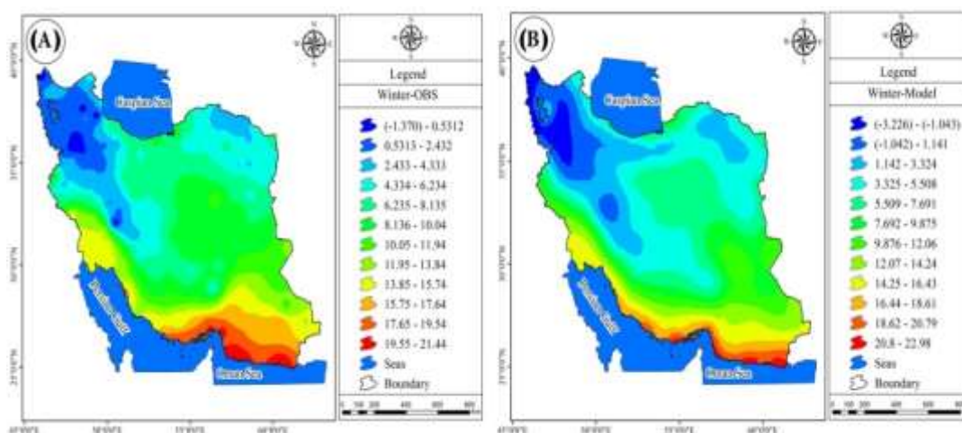
شکل ۳: (A) دمای مشاهداتی (۲۰۱۴-۱۹۸۰) فصل زمستان؛ (B) دمای مدل‌سازی شده (۲۰۵۰-۲۰۱۵) فصل زمستان Figure 3: A) Observed temperature (1980–2014) winter; B) Modeled temperature (2050–2015) winter
