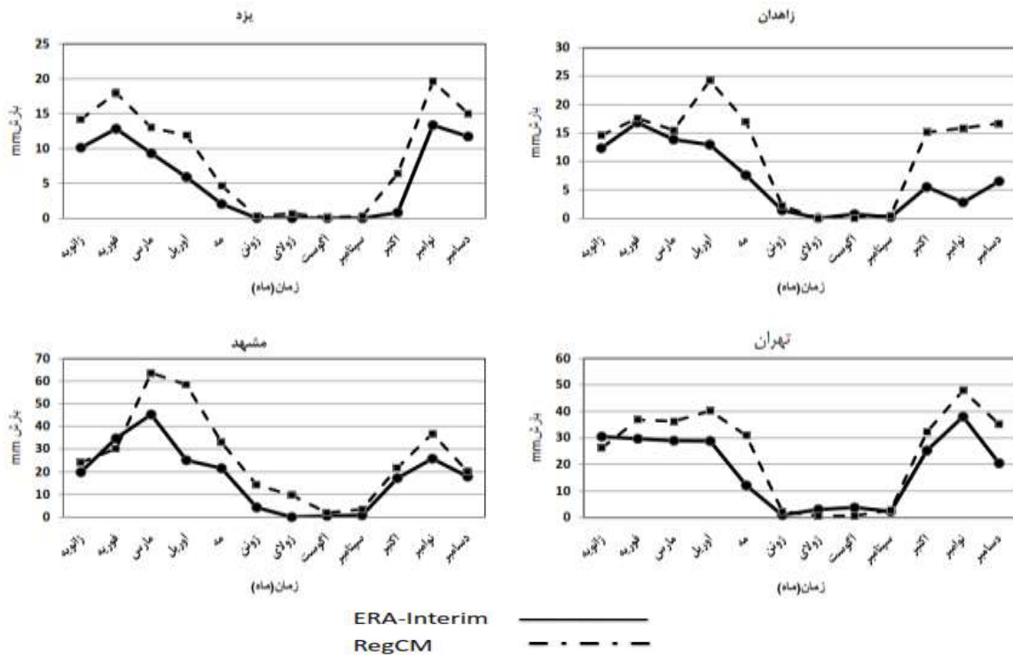
شکل ۴: نمودار میانگین بارش ماهانه تجربی (میلی‌متر) و شبیه‌سازی شده در ایستگاه‌های منتخب در بازه زمانی ۲۰۱۰-۲۰۱۵ Figure 4: Average monthly rainfall graph experimental (mm) and simulated in selected stations in the period 2010-2015
