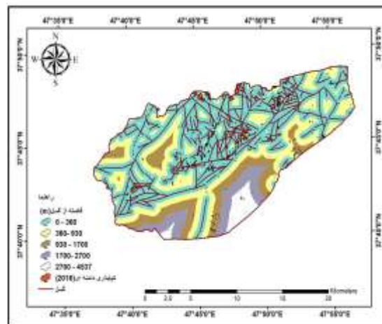
شکل ۶: نقشه فاصله از گسل Figure 6: Distance to fault map
