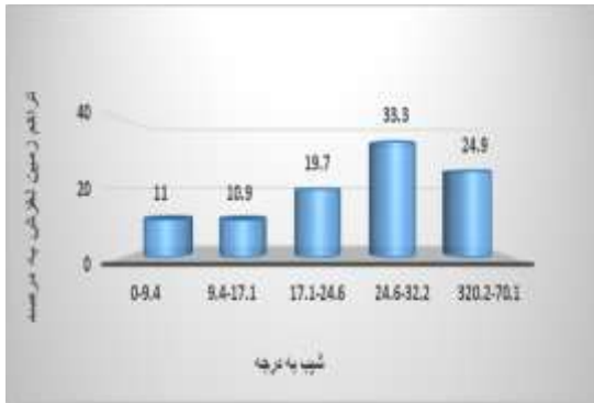
شکل ۱۳: نمودار درصد تراکم ناپایداری دامنه‌ای در کلاس‌های شیب Figure 13: Density percent plot of slope instability for gradient classes
