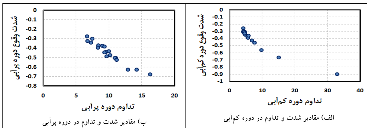
شکل ۲: تغییرات مقادیر شدت وقوع و تداوم در دوره‌های کم‌آبی و پرایبی در ایستگاه‌های هیدرومتری حوزه گرگانرود
