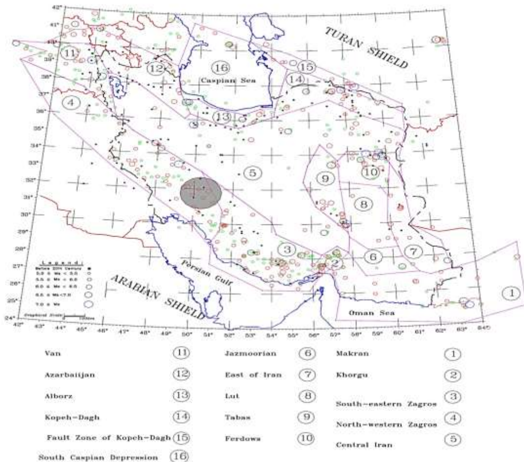
شکل ۳: موقعیت گستره مورد بررسی در نقشه‌ی ایالت‌های لرزه‌زمین‌ساختی ایران بر اساس مدل کمیته ملی سدهای بزرگ ایران (ICOLD,
