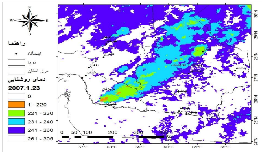
شکل ۴: دمای روشنایی کم‌تر از 260\text{K} باند ۴ سنجنده AVHRR در تاریخ ۲۳ ژانویه ۲۰۰۷ در ساعت 09:52\text{ UTC}
