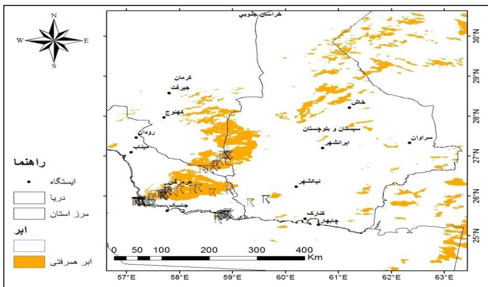
شکل ۱۰: دمای روشنایی کم تر از 240K باند ۴ و بازتابش بیش از ۵۰٪ باند ۲ سنجنده AVHRR در تاریخ ۰۵ ژانویه ۲۰۰۸ ساعت ۶:۵۴ UTC به همراه داده‌های حاصل از سنجنده LIS در ساعت ۷:۳۴ UTC
