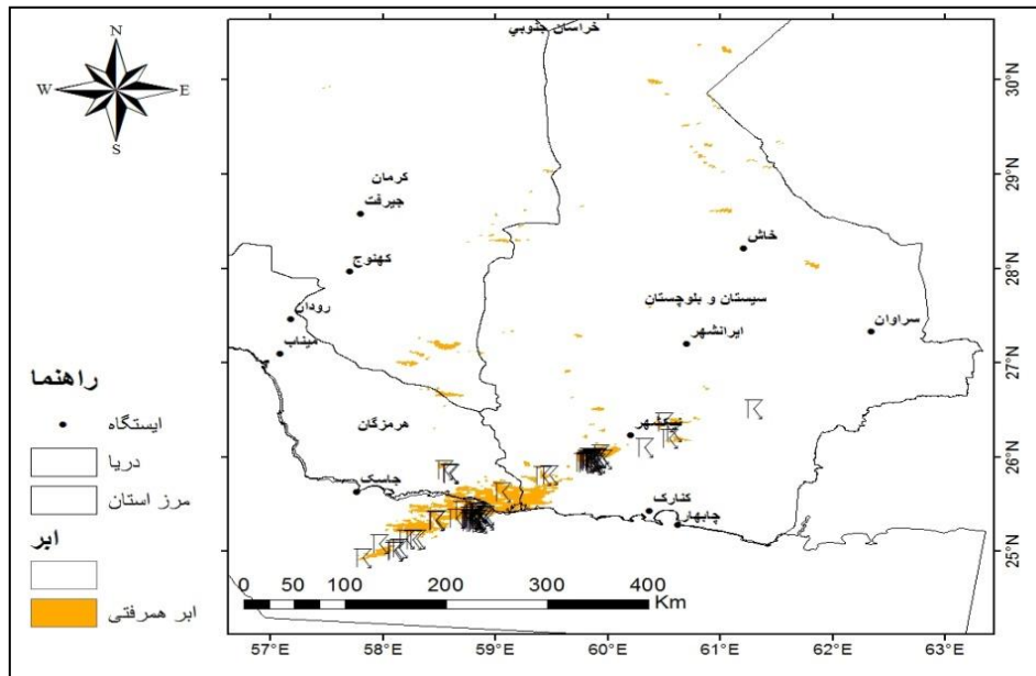
شکل ۹: دمای روشنایی کم تر از 240K باند ۴ و بازتابش بیش از ۵۰٪ باند ۲ سنجنده AVHRR در تاریخ ۱۳ ژانویه ۲۰۰۹ ساعت ۱۰:۰۰ UTC به همراه داده‌های حاصل از سنجنده LIS در ساعت ۱۰:۲۲ UTC
