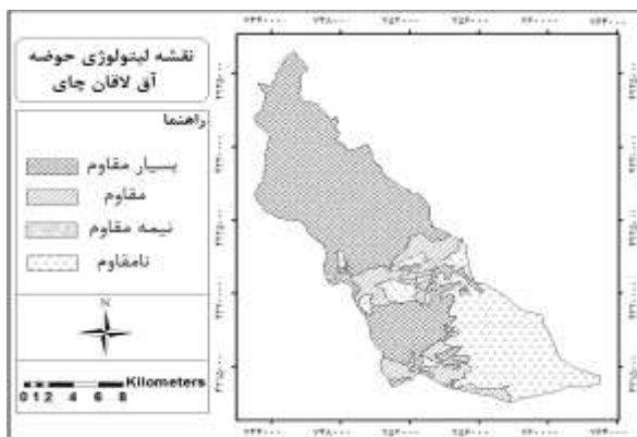
شکل ۵: نقشه لیتولوژی
