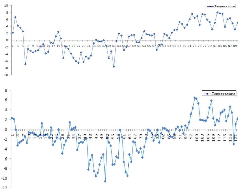
شکل ۳: درجه حرارت‌های ثبت شده برای زمستان سال آبی ۲۰۰۵-۲۰۰۶ (بالا) و سال آبی ۲۰۰۶-۲۰۰۷ (پایین)
