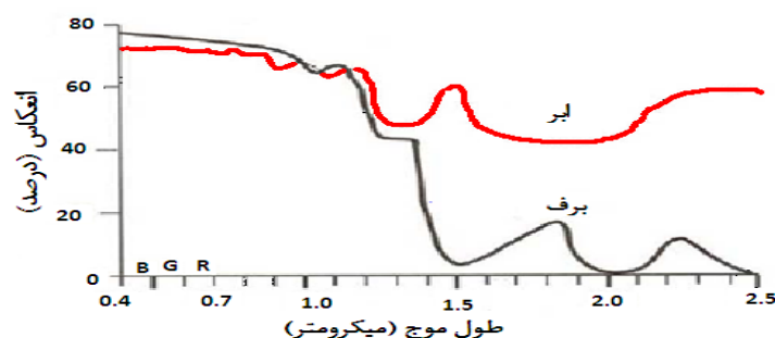
شکل ۲: منحنی انعکاس طیفی برف و یس (جانسون، ۲۰۰۰: ۲)
