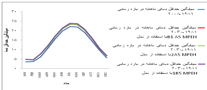
شکل ۱: میانگین حداقل دمای سالانه ثبت شده در ایستگاه رشت طی بازه ۱۹۸۱ تا ۲۰۰۸ و مقادیر پیش‌بینی شده آن برای بازه ۲۰۱۱ تا ۲۰۳۰
