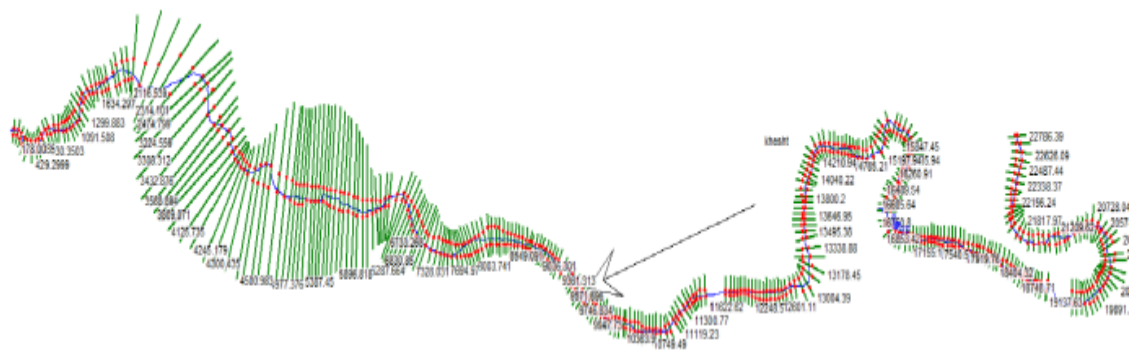
شکل ۱۰: نمای کلی رودخانه‌ی شاپورخشت در مدل هیدرولیکی HEC-RAS
